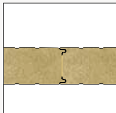
Particolare giunzione
