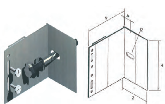
STAFFA NORMALE
