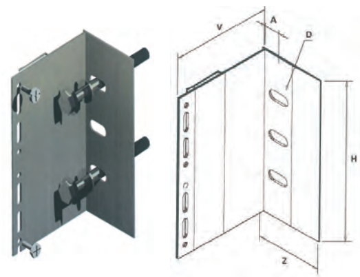
STAFFA LUNGA
