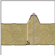
Particolare fissaggio
