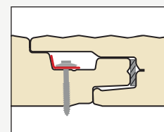
Particolare - Fissaggio nascosto UniWall
