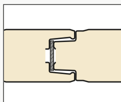
Particolare - Fissaggio a vista
