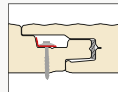
Particolare - Fissaggio nascosto UniWall
